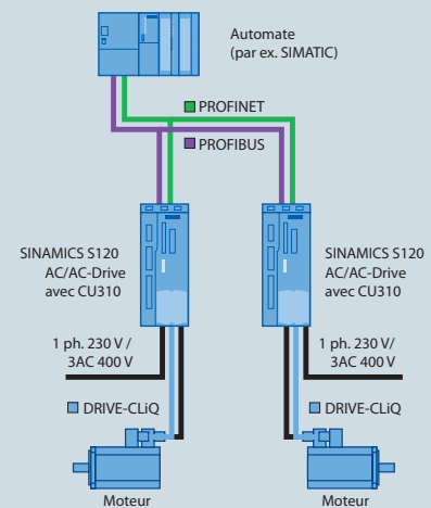
Variateur monoaxe SINAMICS S120 AC/AC
